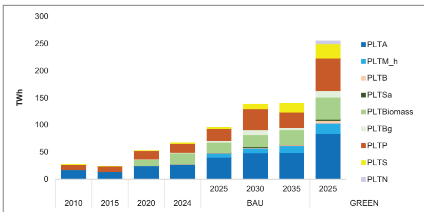
Gambar 3.2 Produksi Listrik EBT per Jenis Pembangkit
