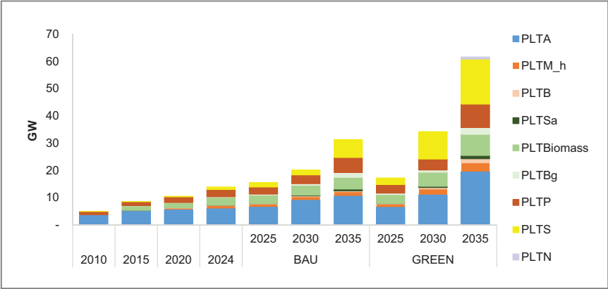
Gambar 3.5 Kapastias Pembangkit Listrik EBT per Jenis Pembangkit
